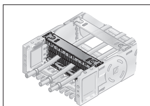
Щеточный держатель
